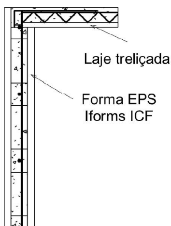
Figura 6 – Interface entre parede e laje
