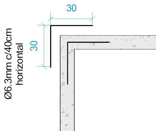
Figura 5 – Ligação entre paredes a 90 graus
