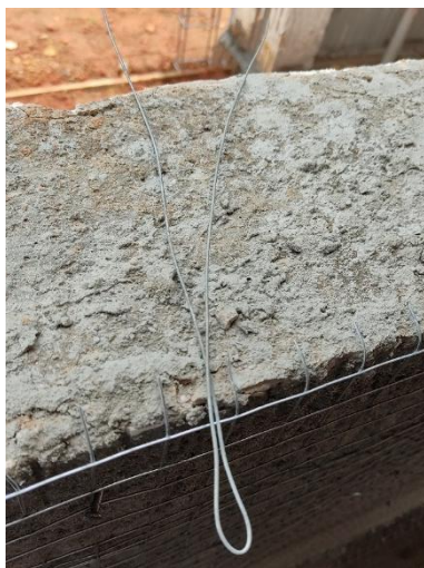
Figura 23 – Conector das telas do revestimento
